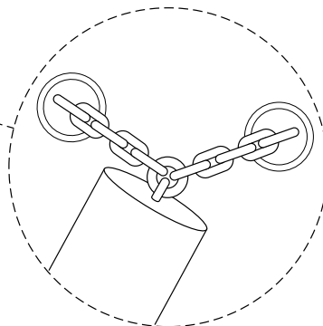
DETALLES DE LOS ANILLOS OCULARES Y SISTEMAS DE PROTECCIÓN CON CADENA INTEGRADA
