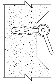
SECCIÓN TRANSVERSAL DEL ALOJAMIENTO DEL PERNO INTEGRADO EN HORMIGÓN
