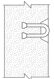
SECCIÓN TRANSVERSAL DEL ALOJAMIENTO DEL ANILLO OCULAR INTEGRADO EN HORMIGÓN
