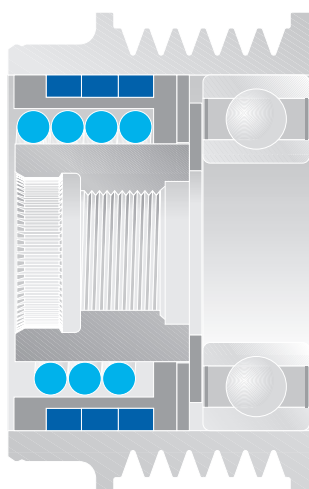
Polea libre del alternador desacoplada (Overrunning Alternator Decoupler - OAD)
